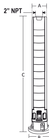
Acoplamiento NEMA 4"
